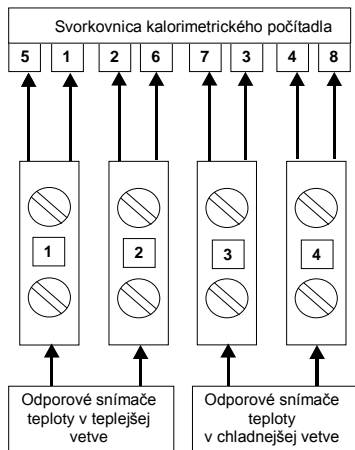
Obr.: 6 Pripojenie káblov odporových snímačov teploty
