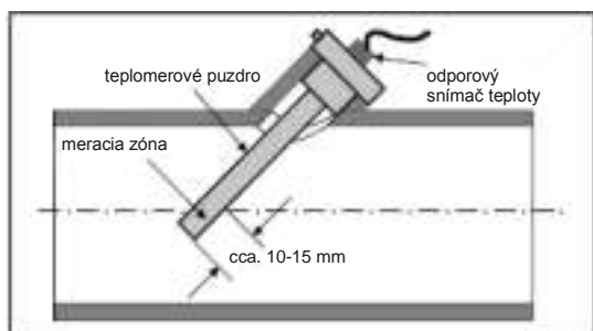
Obr.4 Príklad montáže merača veľkosti \leq DN 80
