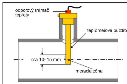
Obr.. 5: Príklad montáže merača veľkosti DN 100
