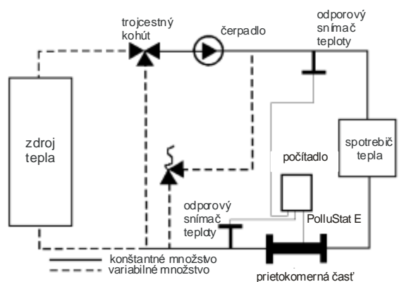
Obr. 3: Systém s prepadovým ventilom
